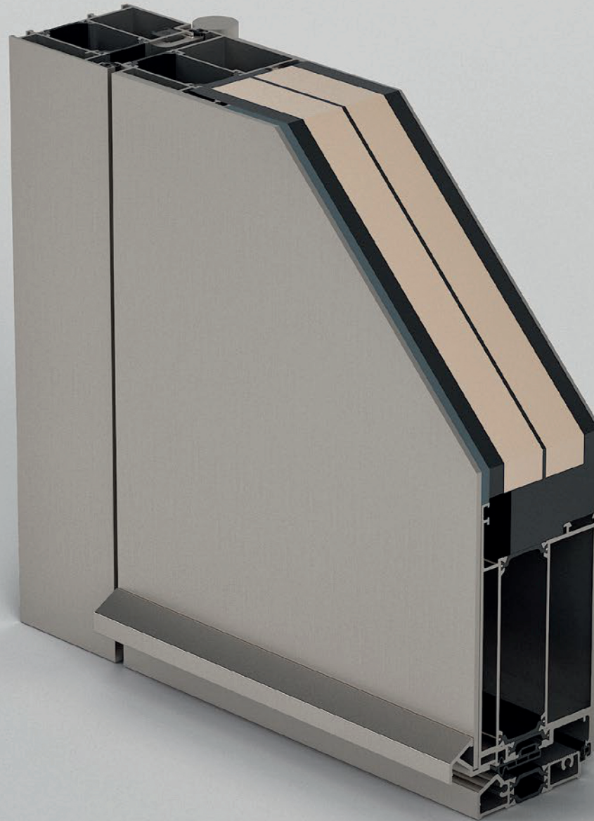
Esploso 3D Sezione senza fermavetro
