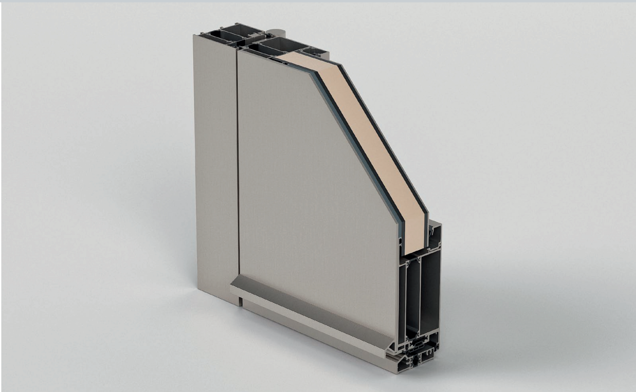
Esploso 3D Sezione con femavetro
